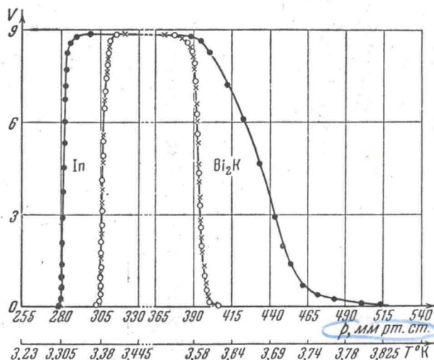
Рис. 1. Смещение T_k \text{Bi}_2\text{K} с давлением. Слева приведено градуировочное смещение индия; \circ — образец без давления, \bullet — давление p = 1520 \text{ кг/см}^2 , \times — давление снято. T_k определяется из середины кривых перехода
